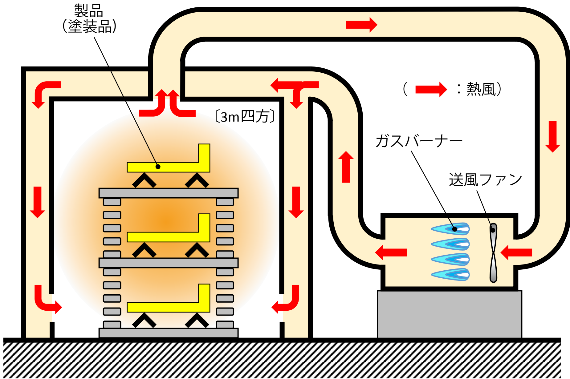
金庫型熱風乾燥炉構造図
