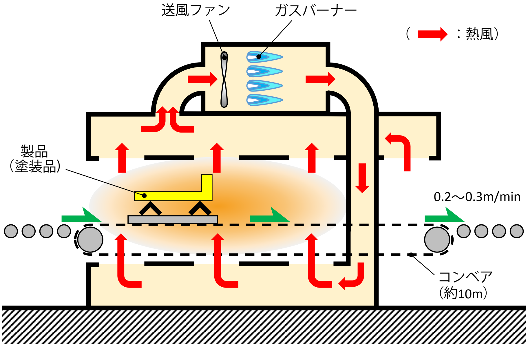
コンベア型熱風乾燥炉構造図
